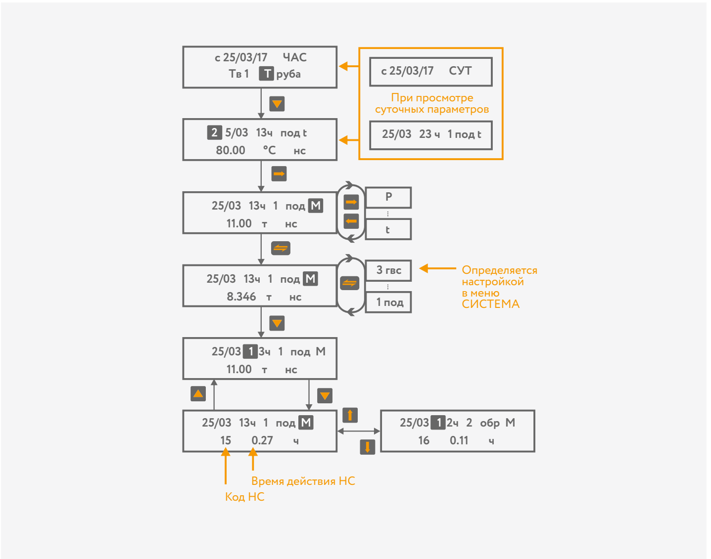
Рисунок 23 – Просмотр архивной информации по кодам и времени действия НС
