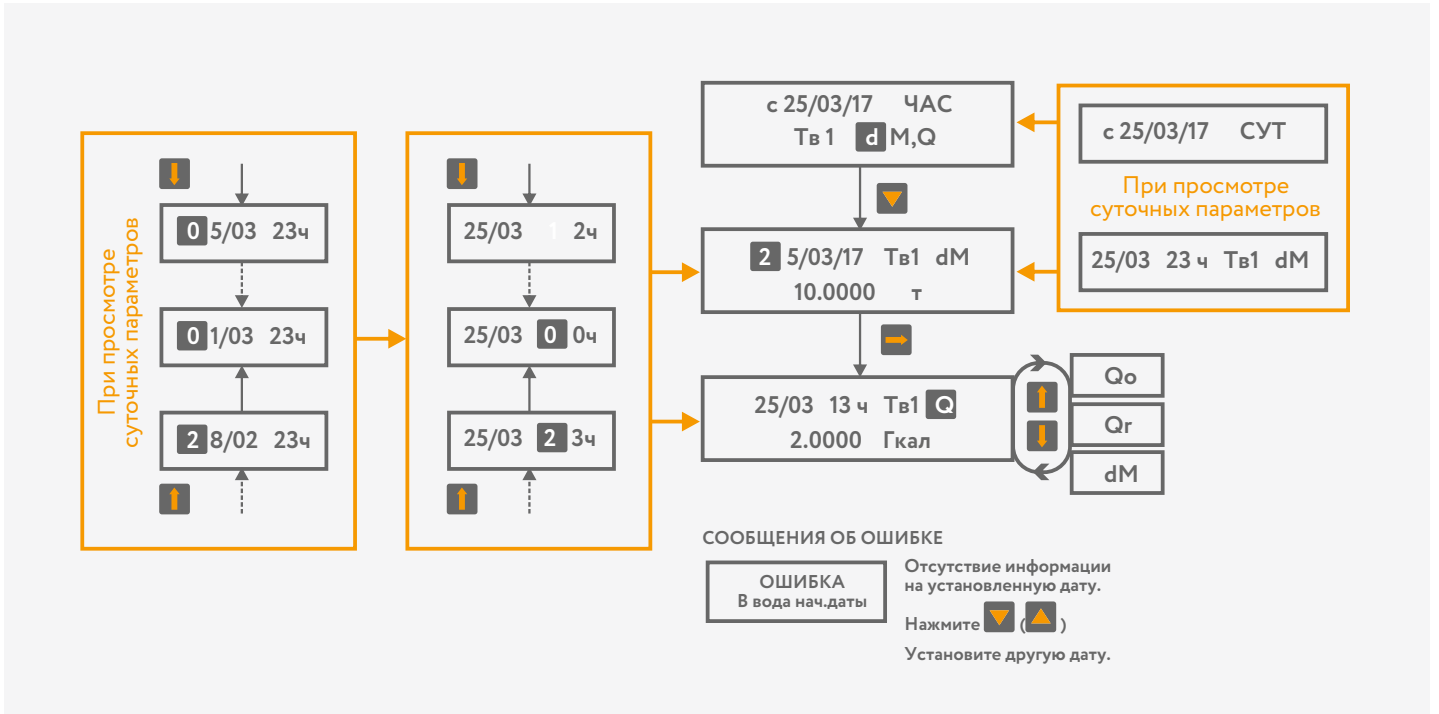
Рисунок 20 – Просмотр архивной информации по тепловому вводу
