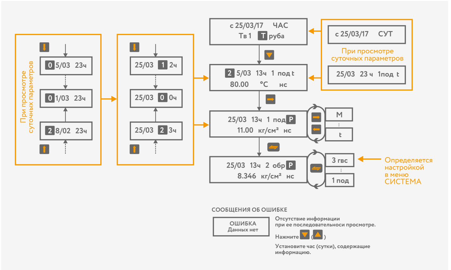
Рисунок 21 – Просмотр архивной информации по трубопроводу
