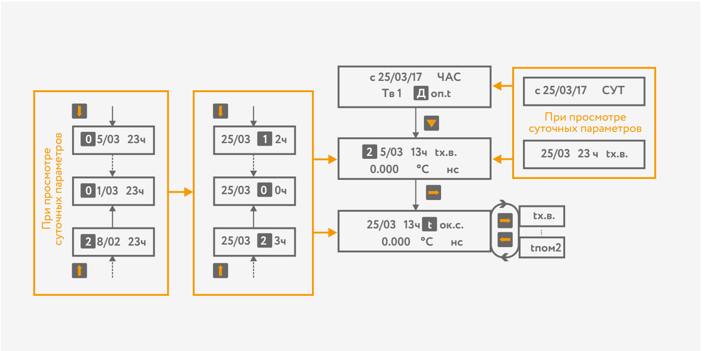
Рисунок 22 – Просмотр архивной информации по температуре среды
