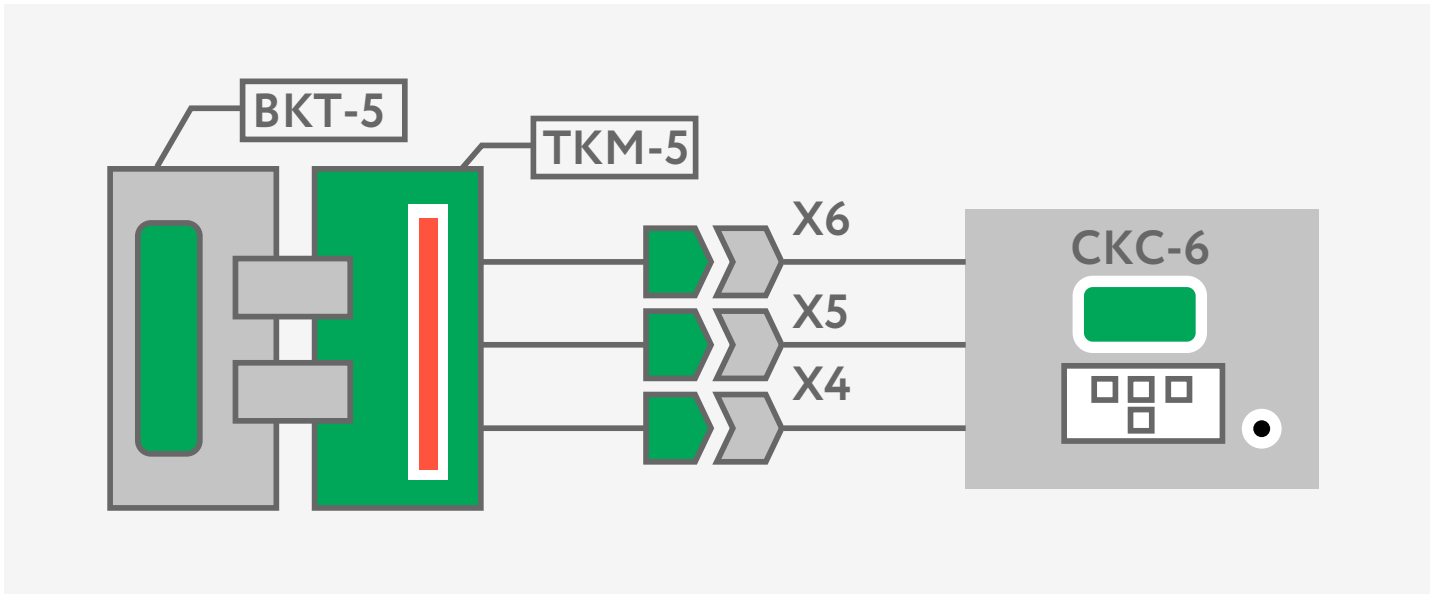
Рис. Б.2 Схема поверки ВКТ-5 с использованием СКС-6 и ТКМ-5 Разъемы X4...X6 (ТКМ-5) подключаются к одноименным разъемам стенда СКС6
