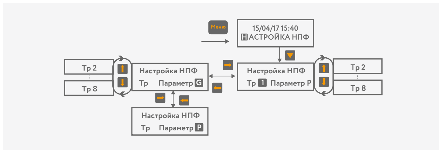
Рисунок 6.1 – Последовательность действий по настройке НПФ датчиков давления и расхода.
