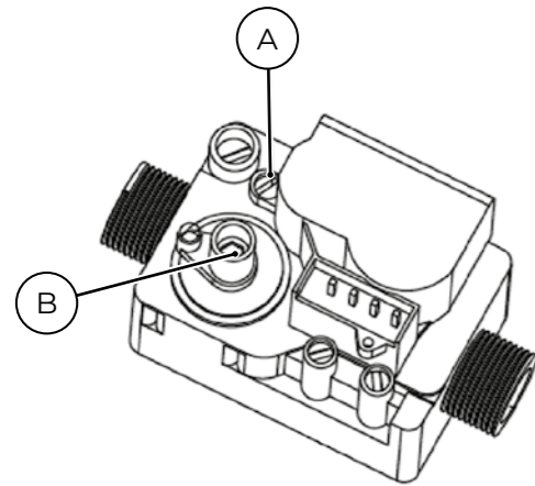
Рис. 19. Газовый клапан.
