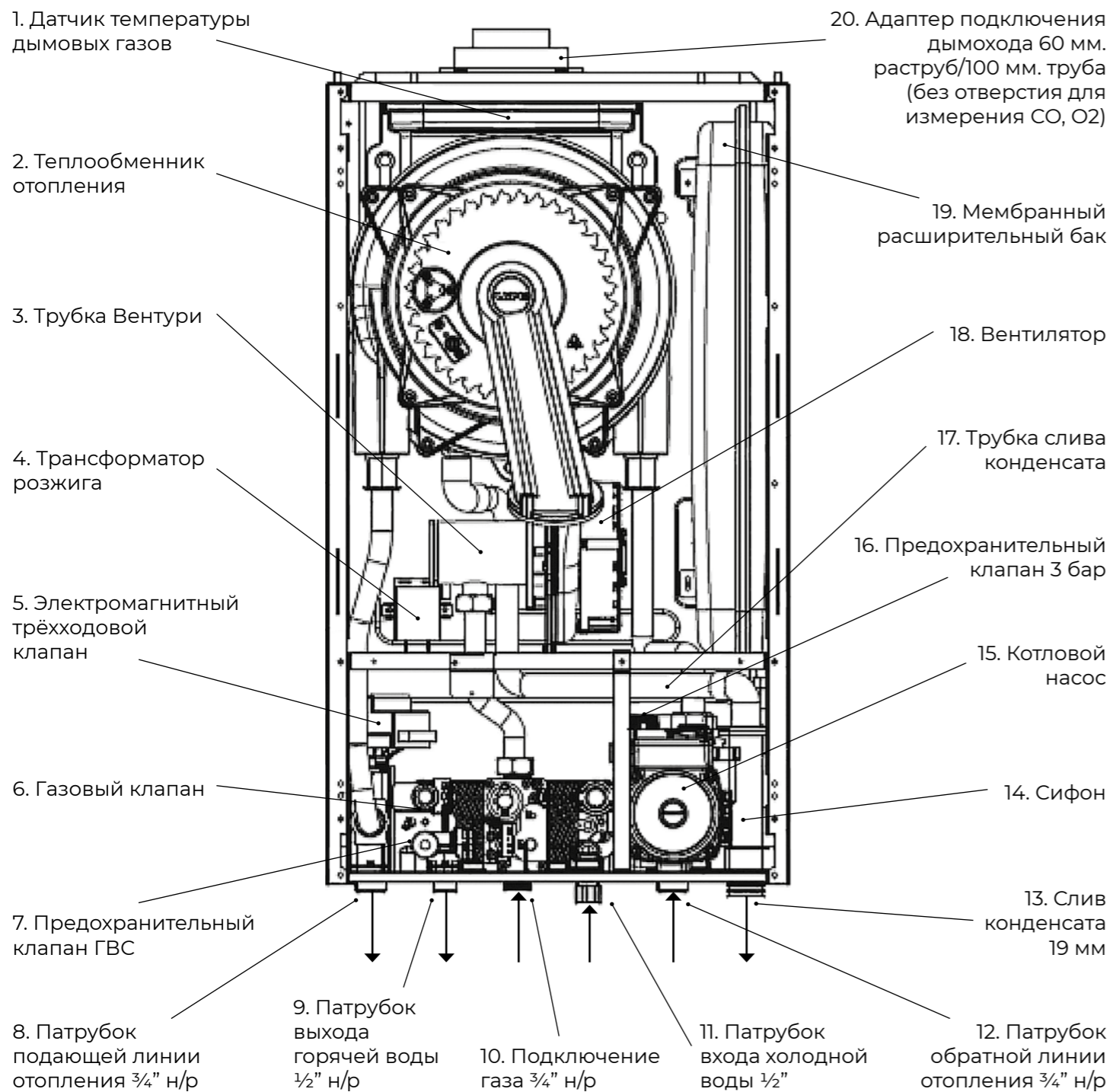
Рис. 2. Общая схема.
