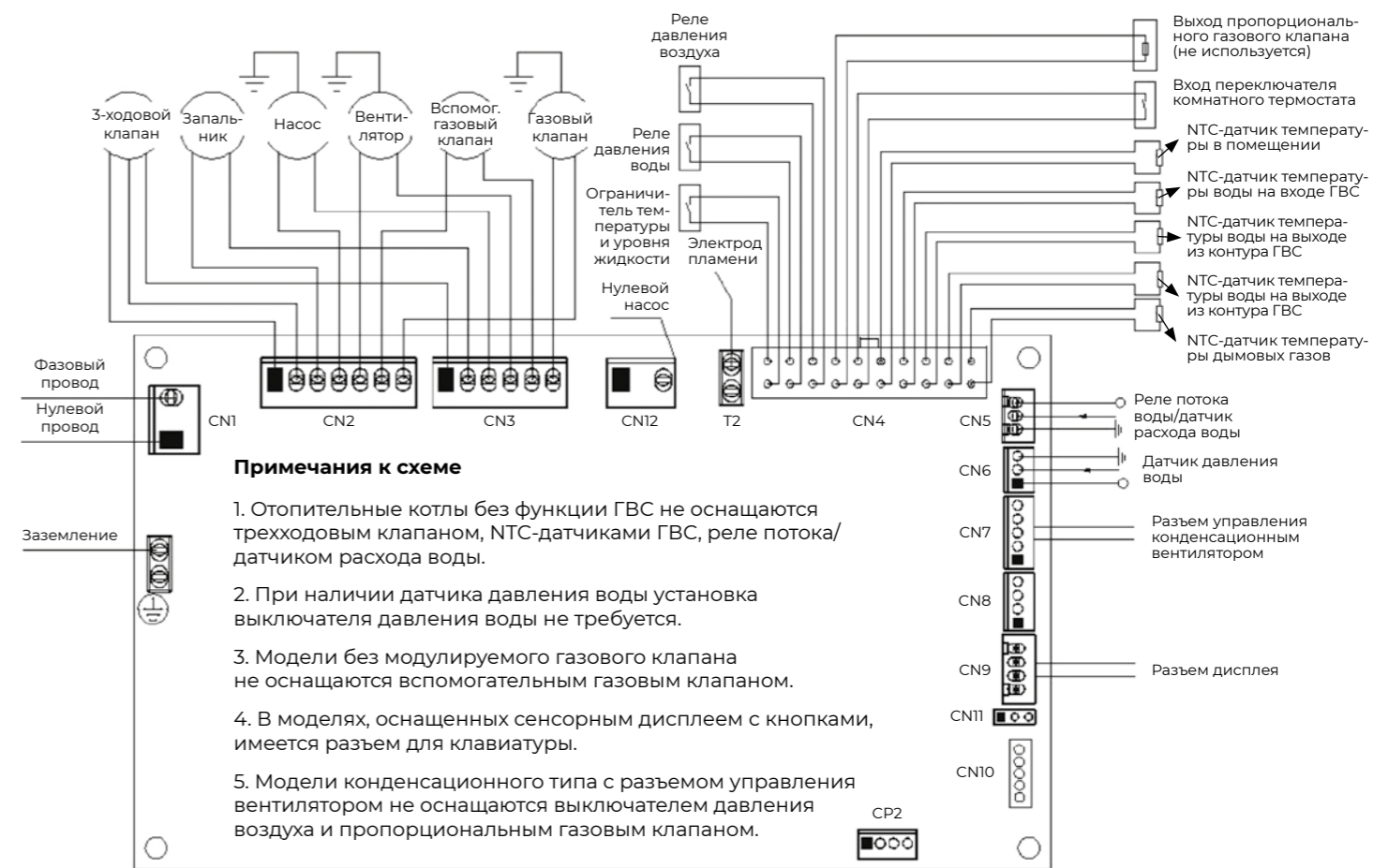
Рис. 26. Электрическая схема.
