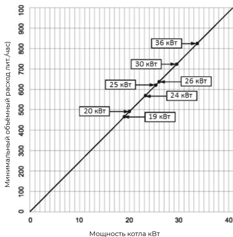
Диаграмма 5. Минимальный объемный расход через котёл.
