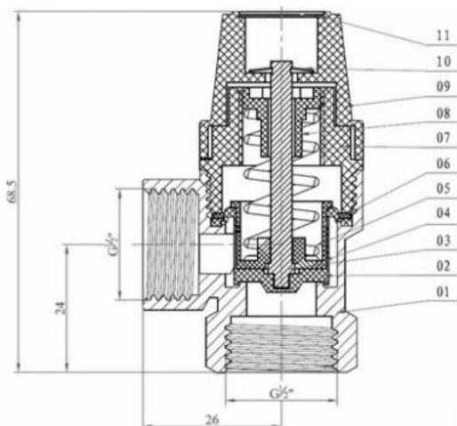
Рис.1. Клапан предохранительный DN15×15 BP.
