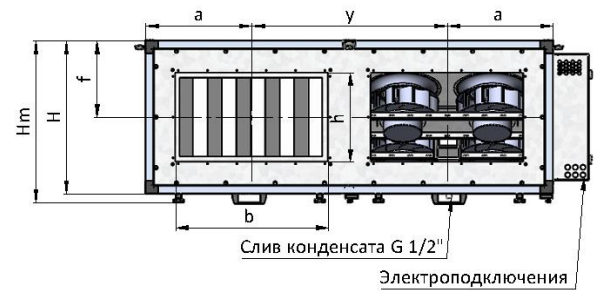
Вид слева
