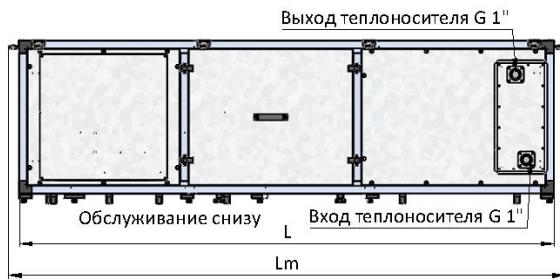
Вид спереди
