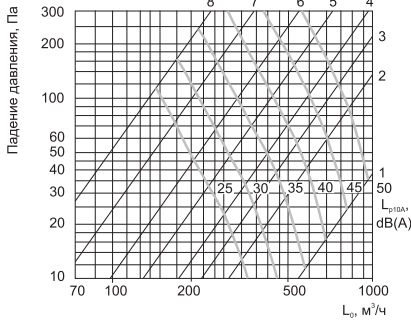
IRIS (SS316)-315
