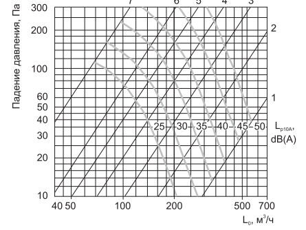
IRIS (SS316)-125
