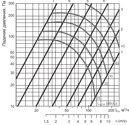
IRIS (SS316)-160
