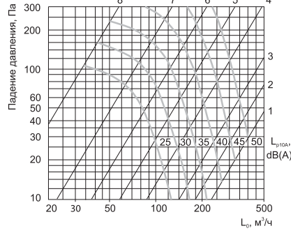
IRIS (SS316)-100
