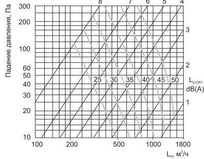
IRIS (SS316)-400
