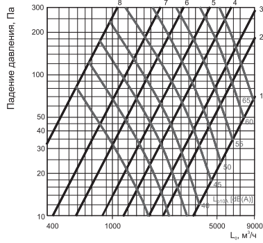
IRIS (SS316)-800
