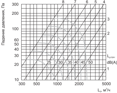
IRIS (SS316)-315
