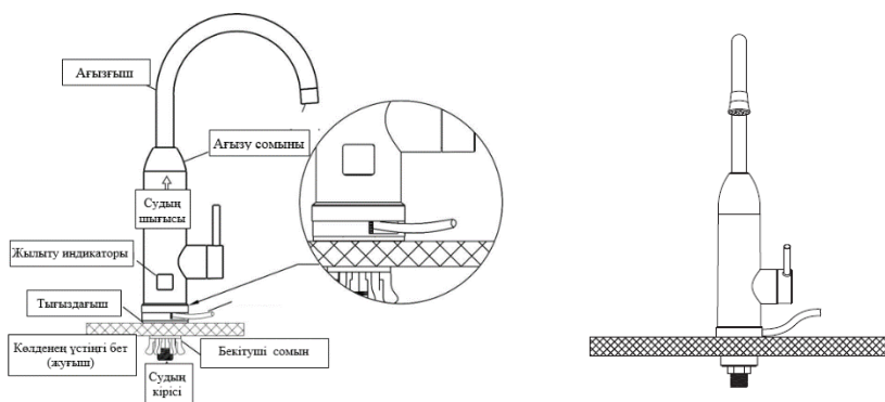
2-сур. Қорек беру кабелін жуғыштың астынан шығарумен орнату
