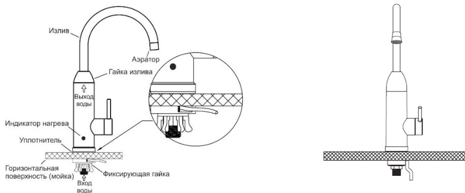
Рис. 2. Установка с выводом кабеля питания под мойкой
