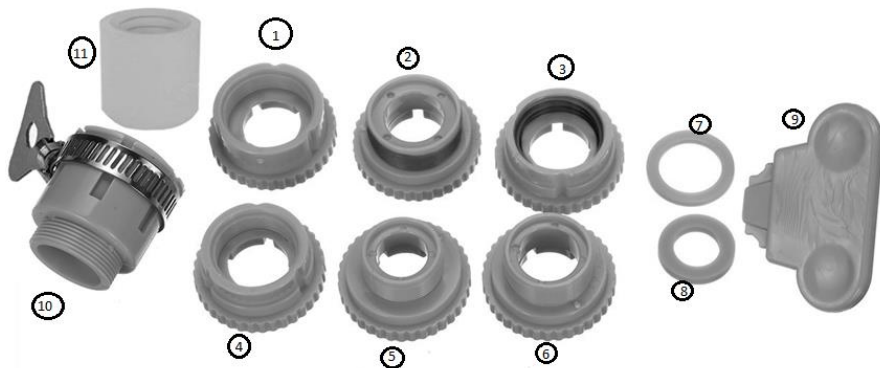
Рис.1. Монтажный комплект:
