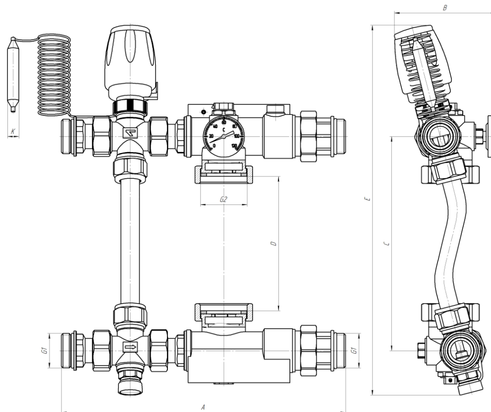
Рисунок 4 – Габаритные и присоединительные размеры изделия
