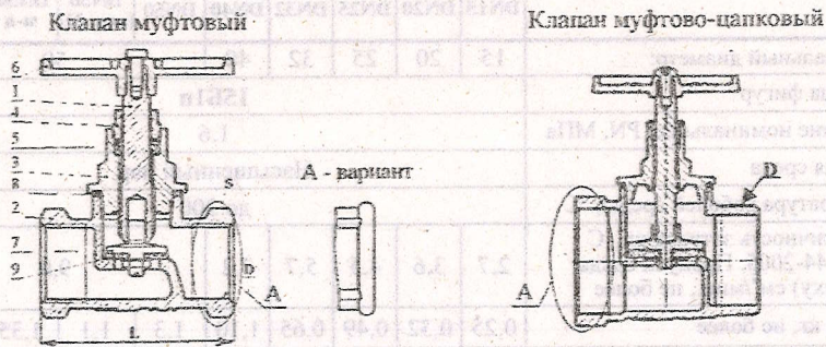
1 - шпindelь; 2 - корпус; 3 - крышка; 4 - гайка сальника; 5 - втулка сальника; 6 — маховик; 7 - золотник; 8 - прокладка; 9 - прокладка золотника.
